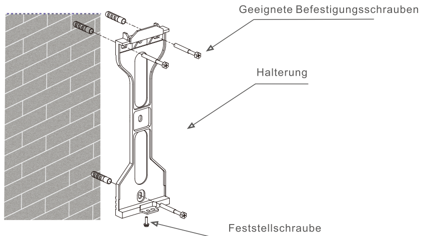
Abbildung 4.4 Halterung an der Wand befestigen
