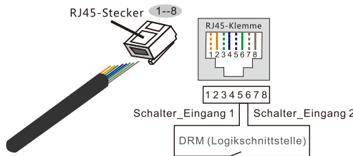
Abbildung 4.13 Die Isolierung entfernen und sie an den RJ45-Stecker anschließen
