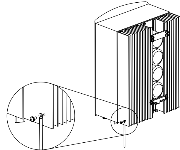
Abbildung 4.11 Den externen Erdungsleiter anschließen
